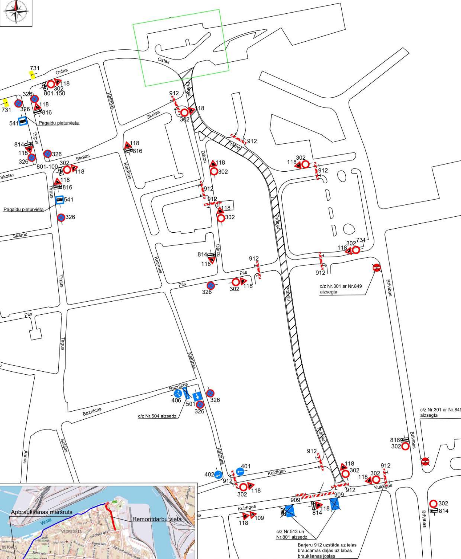
Satiksmes organizācijas shēma Prāmja ielas pārbūvei (no Kuldīgas ielas līdz Ostas ielai), Ventspilī. Ceļa zīmju izvietojumu shēma.
